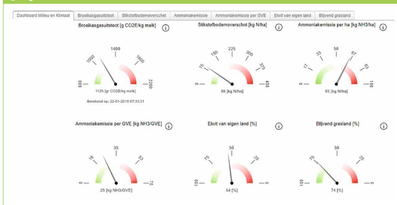
Figuur 6. Dashboard Milieu en Klimaat
